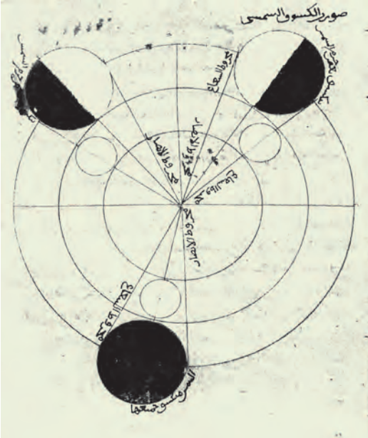
Διάγραμμα πηλίκης έκλειψης από χειρόγραφο του al-Karkhi, 11ος αιώνας μ.Χ.
